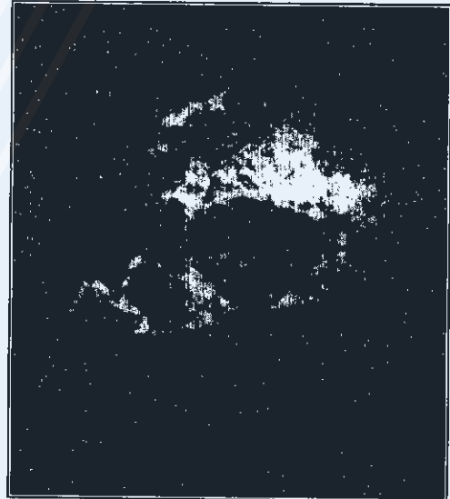
يرى هنا سديم الوردية في صورة التقطها مرصد شميت في مرصد بالومار، ويقع السديم في كوكبة وحيد القرن.
