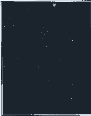
سديم رأس الفرس، على مقربة من زيتا الجوزاء.
