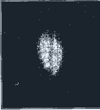
المرأة المسلسلة، وهي وراء مجرتنا، تبعد عنا (٢,٢) مليون سنة ضوئية.
