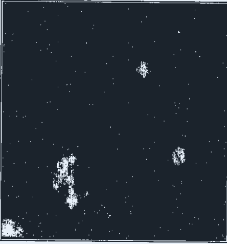
السديم المظلم يفسّي ضوء النجوم الموجودة وراءه وخير مثال على ذلك كيس الضم.
